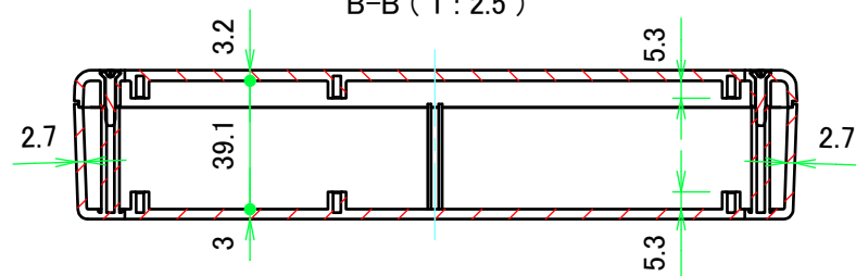
B-B ( 1 : 2.5 )
