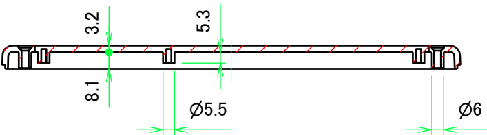
D-D ( 1 : 2.5 )
