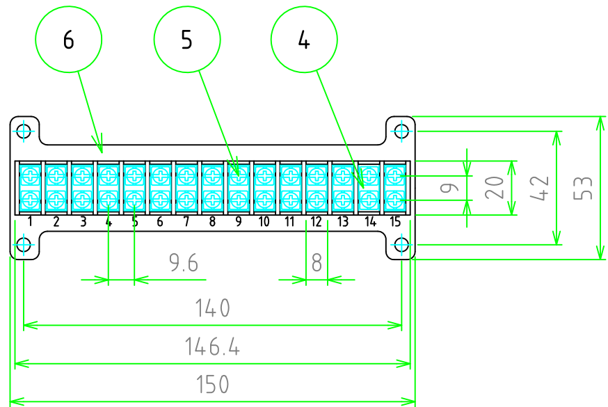
端子台詳細図
