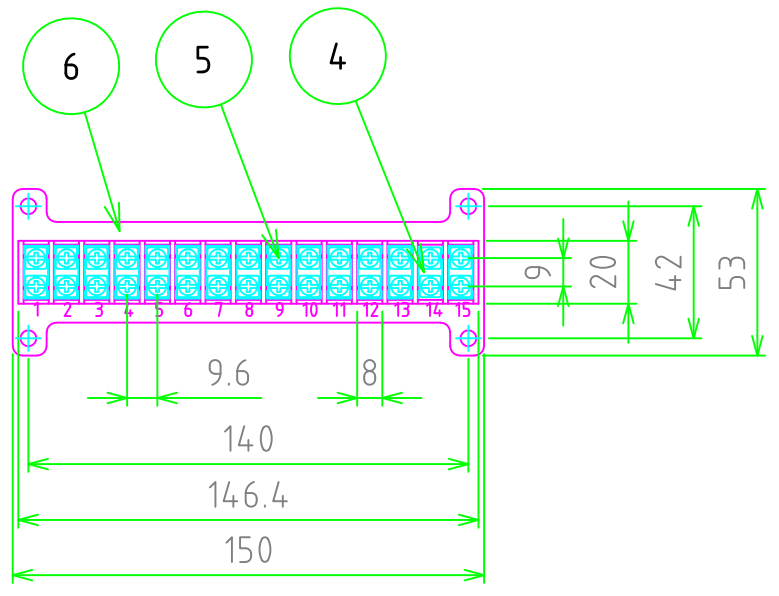
端子台詳細図
