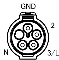
プラグ側
