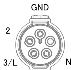
ソケット側
