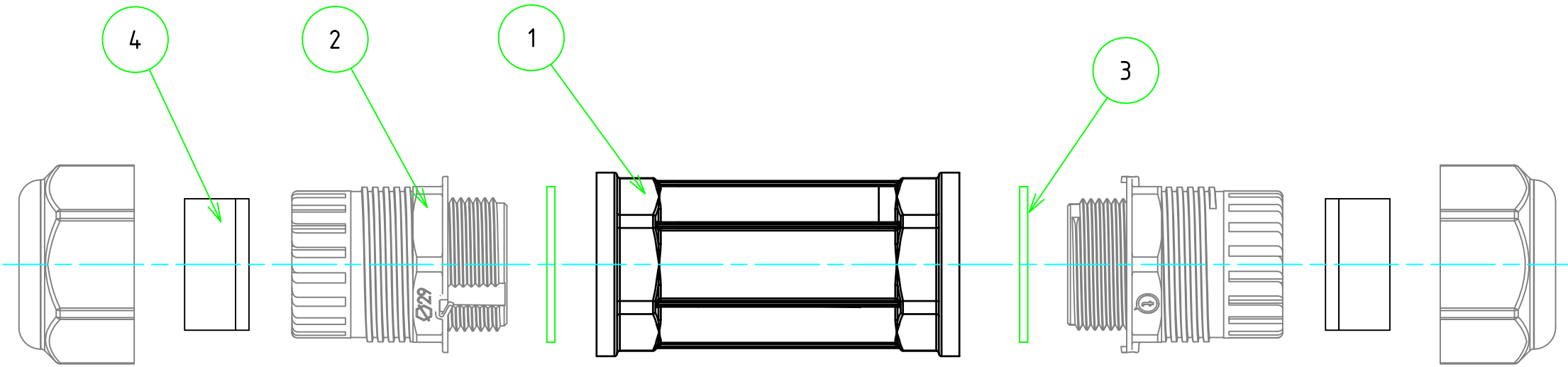
展開図
