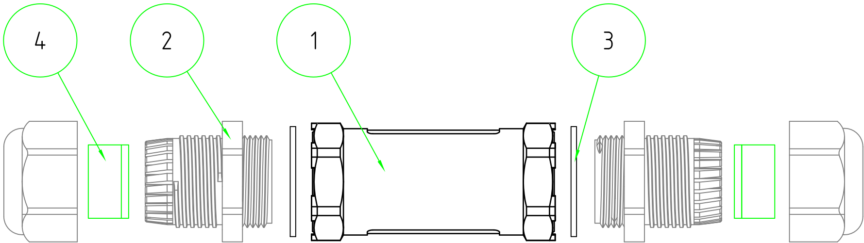
展開図
