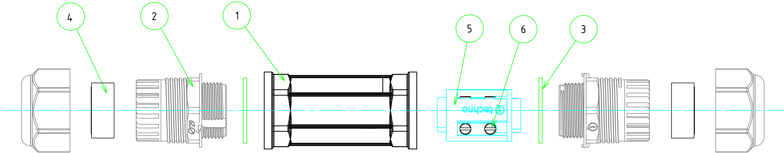
展開図
