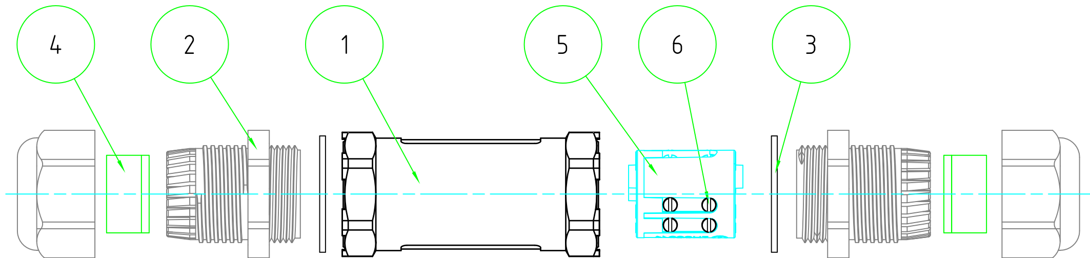
展開図
