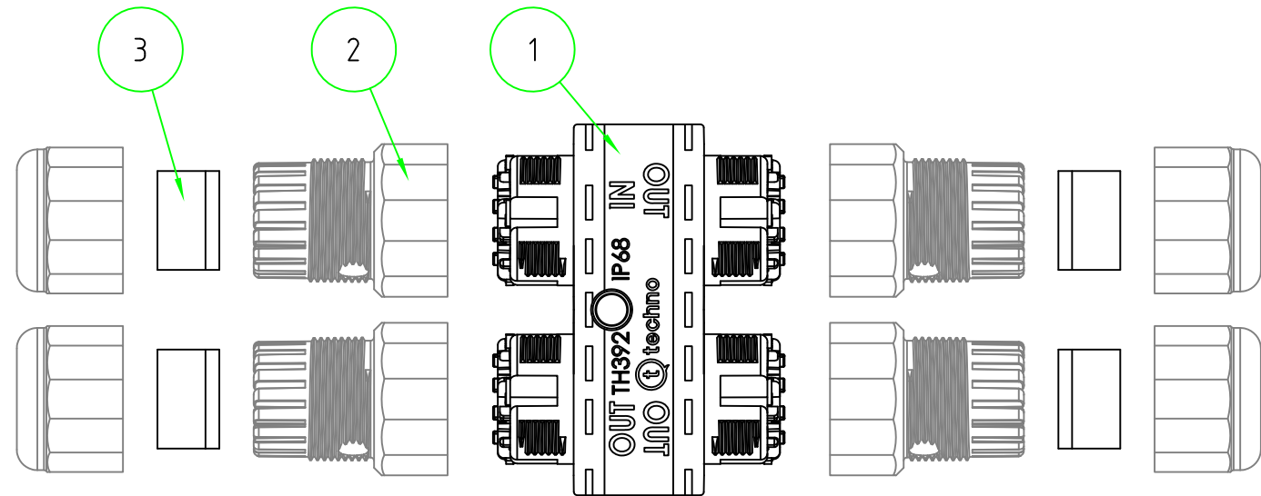
展開図
