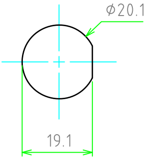
取付穴寸法
