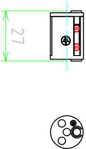
3P 端子台
