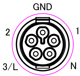
プラグ側
