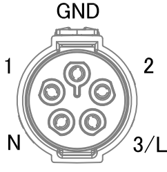
ソケット側
