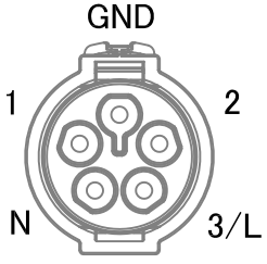
プラグ側
