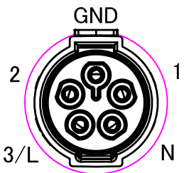
ソケット側
