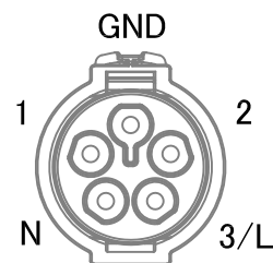
プラグ側
