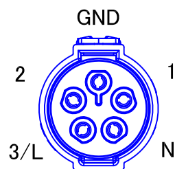
ソケット側
