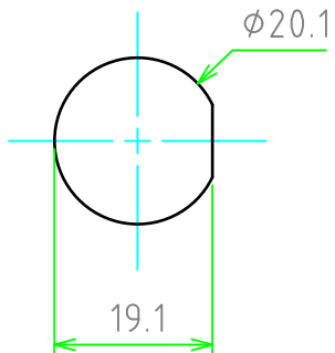
取付穴寸法
