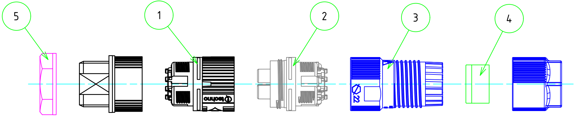
展開図
