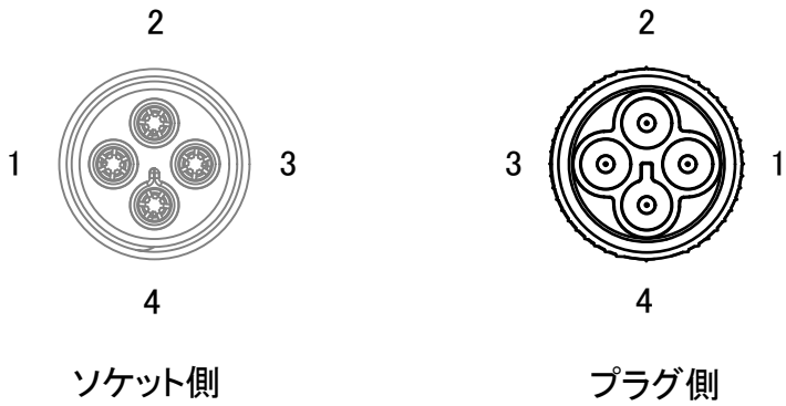
端子配列図
