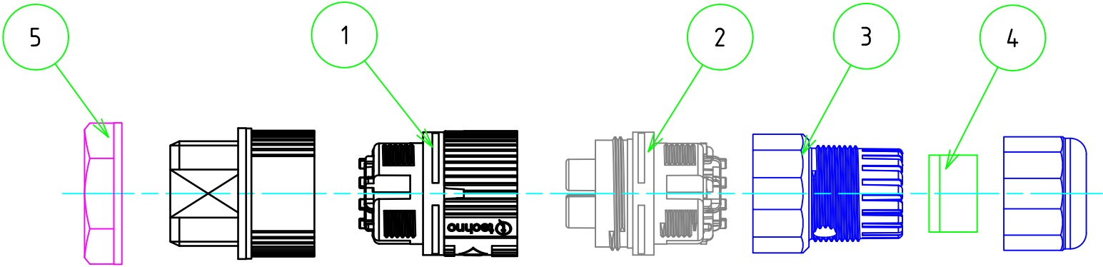
展開図
