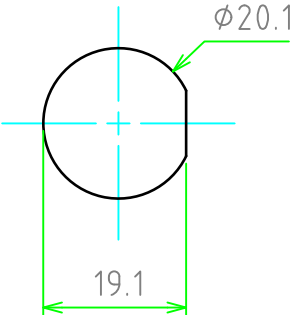
取付穴寸法
