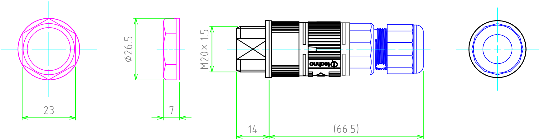
展開図
