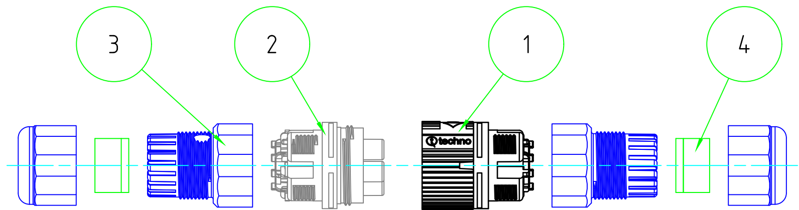
展開図
