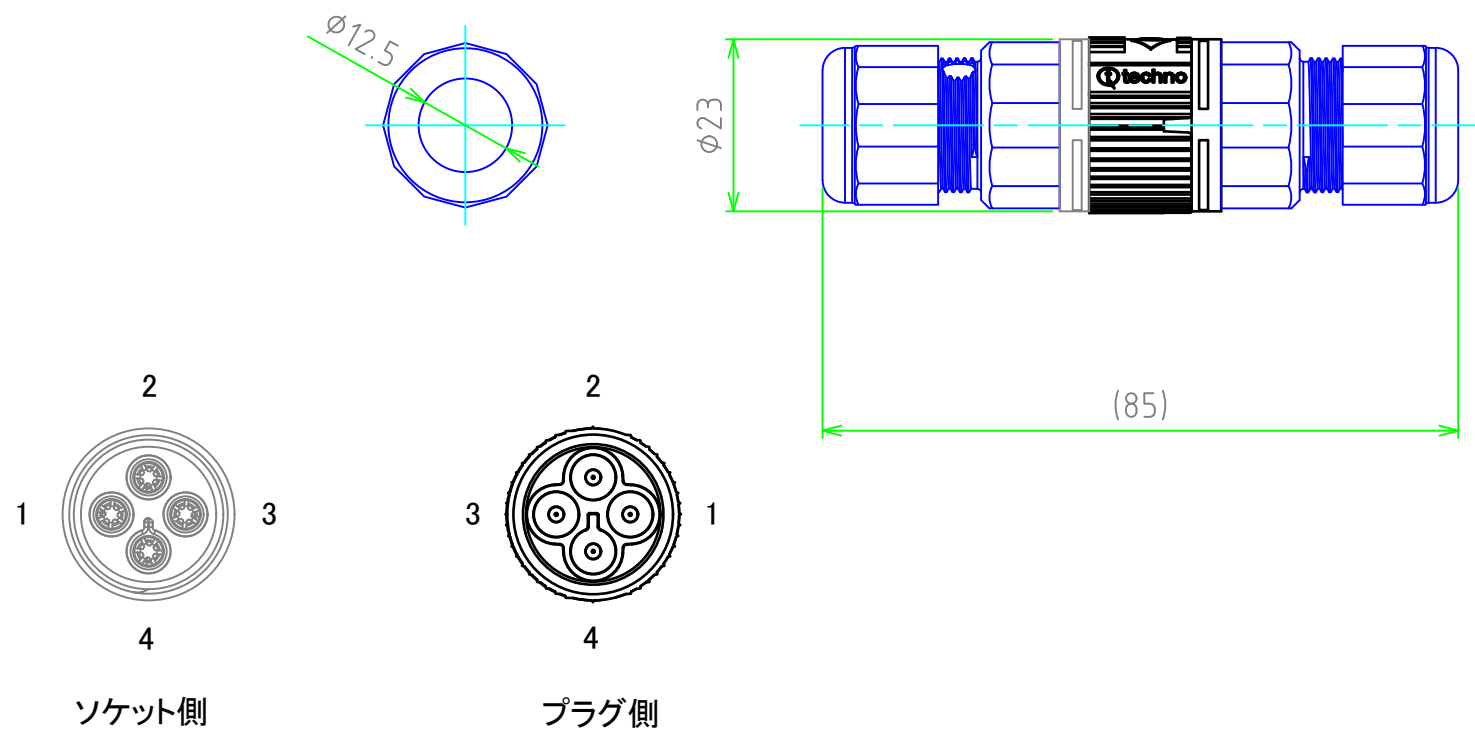
端子配列図
