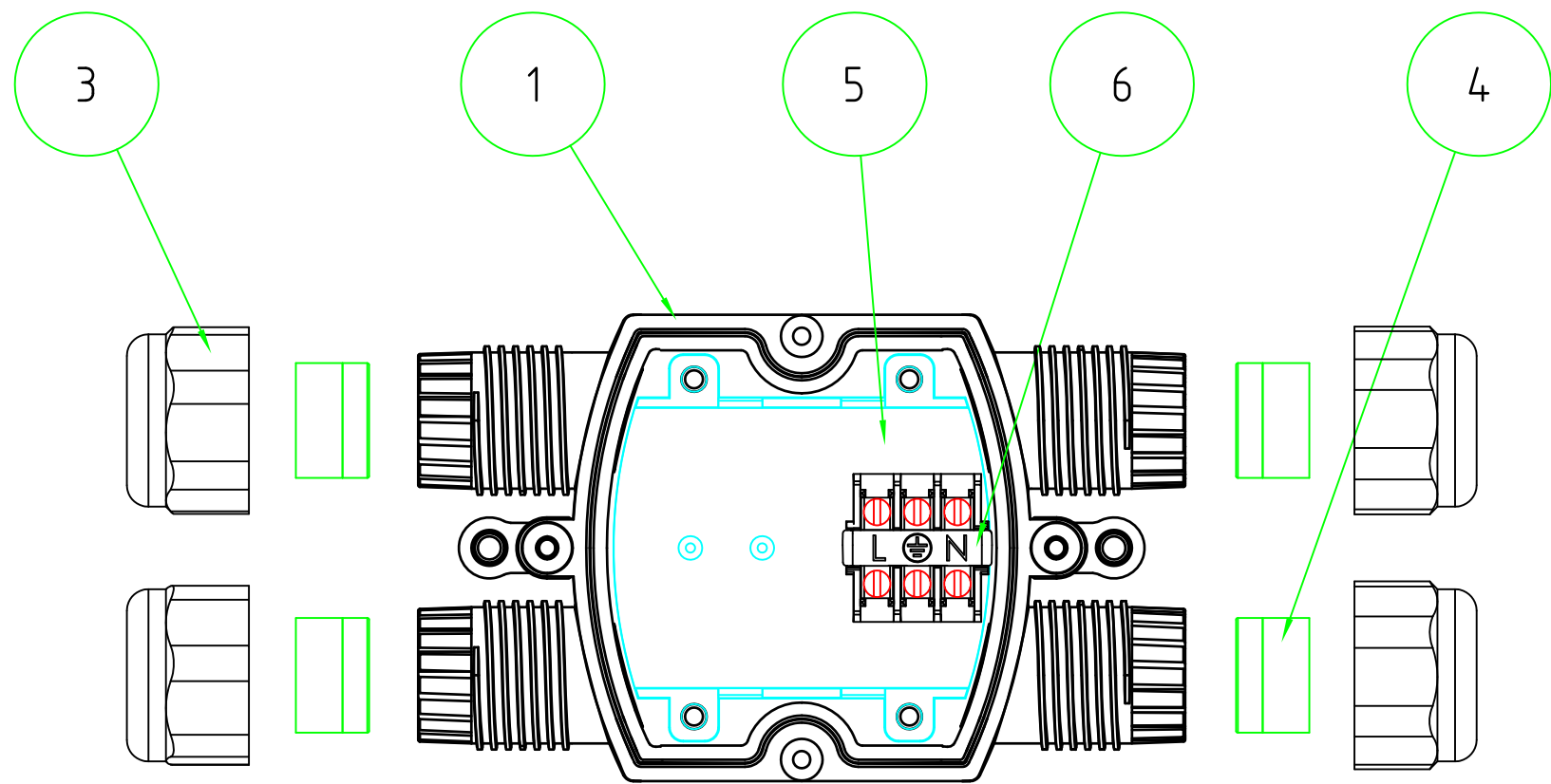
展開図
