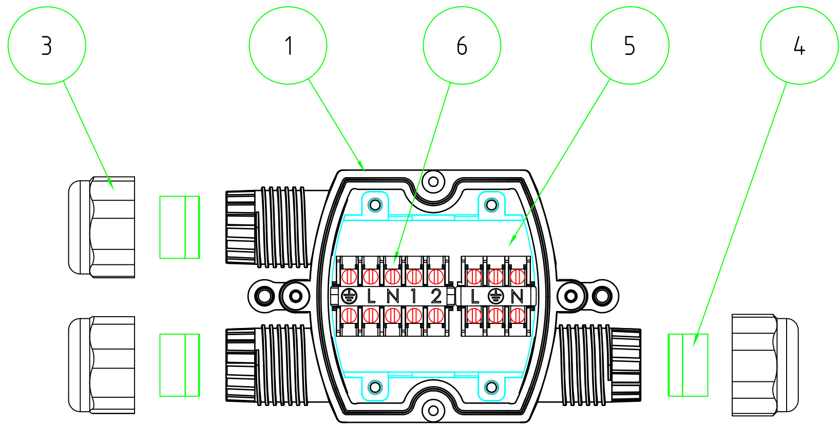
展開図
