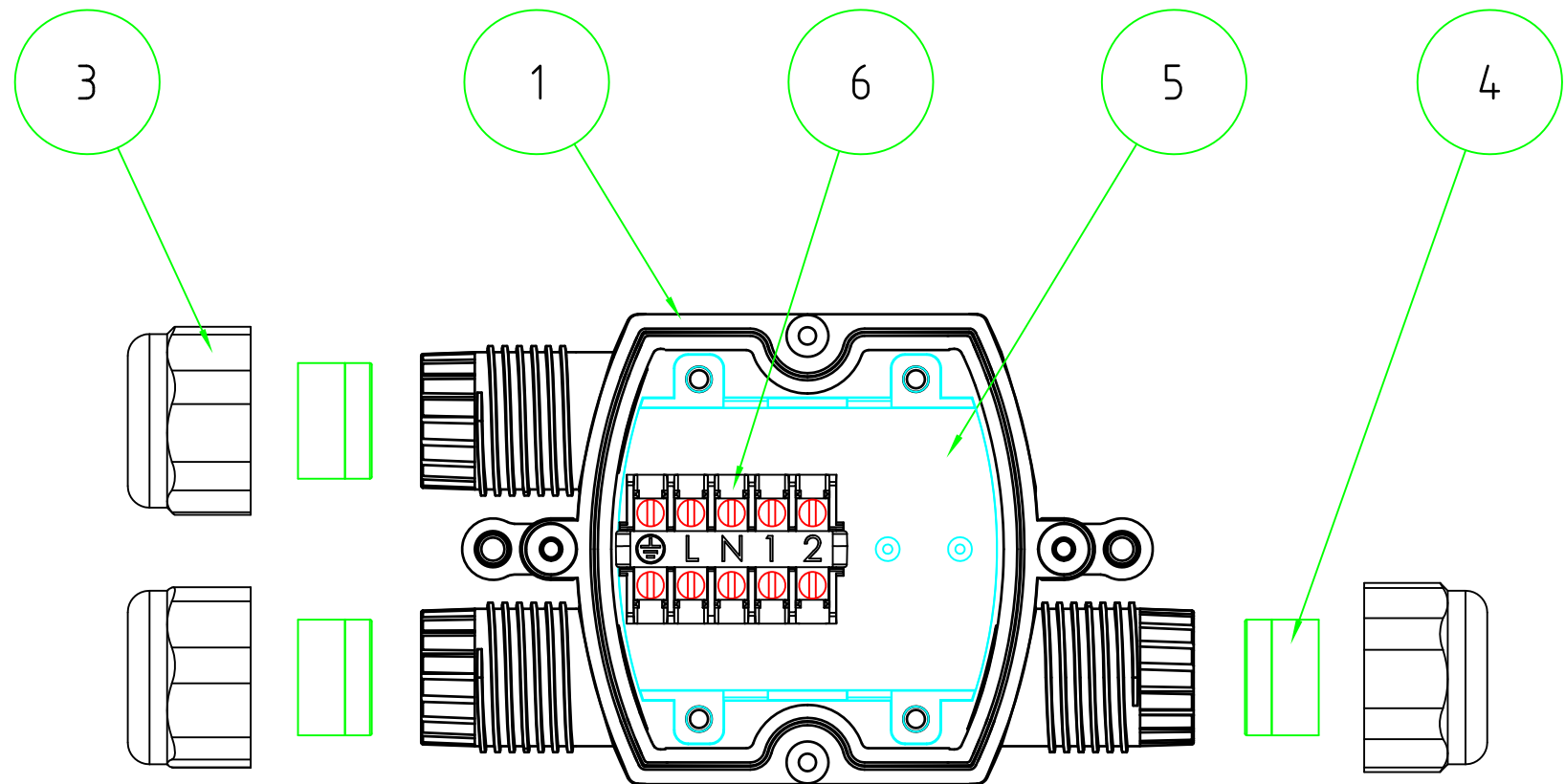
展開図
