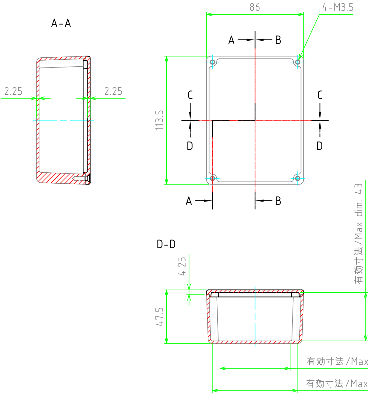
ボディー(内視) Base (Internal View)
