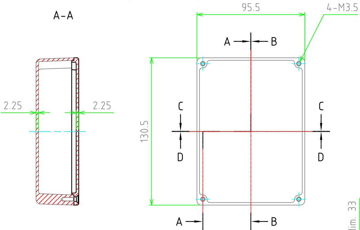
ボディー(内視) Base (Internal View)
