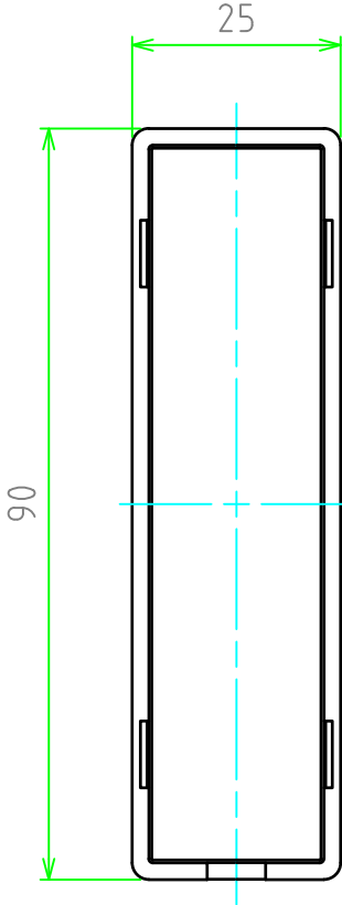
ボディー (内視) Base (Internal View)
