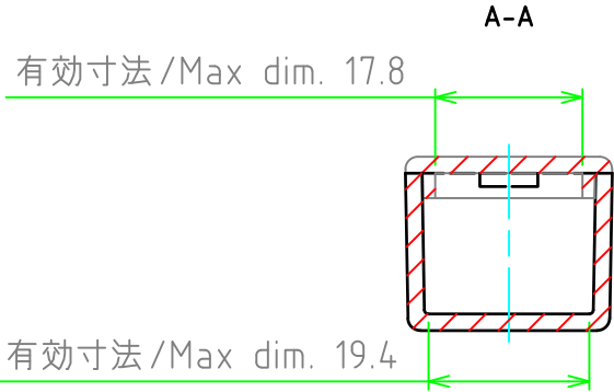
カバー (内視) Cover (Internal View)
