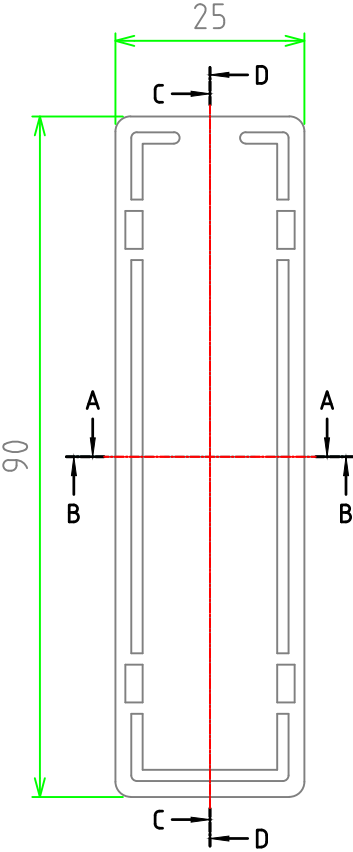
カバー (内視) Cover (Internal View)
