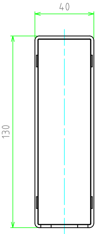
ボディー (内視) Base (Internal View)
