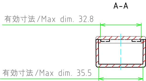
カバー (内視) Cover (Internal View)
