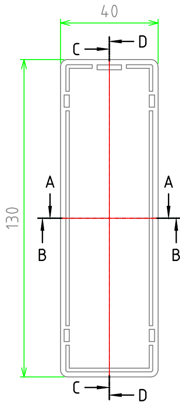
カバー (内視) Cover (Internal View)
