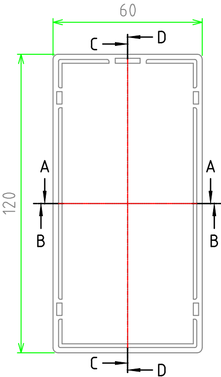
カバー (内視) Cover (Internal View)
