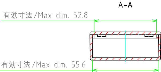
カバー (内視) Cover (Internal View)
