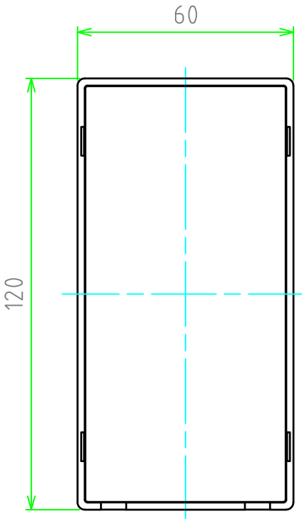
ボディー (内視) Base (Internal View)
