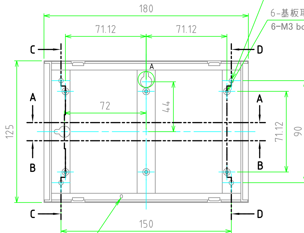
ボディー (内視) Base (Internal View)
