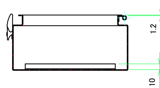
A-A ( 1 : 4 )
