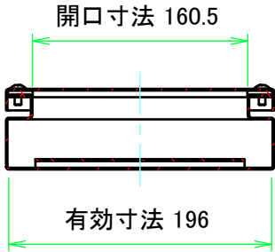
A-A ( 1 : 5 )
