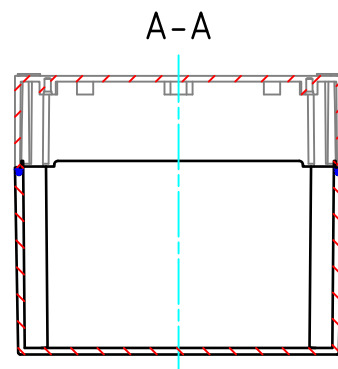
ボディー(内視) Base (Internal View)
