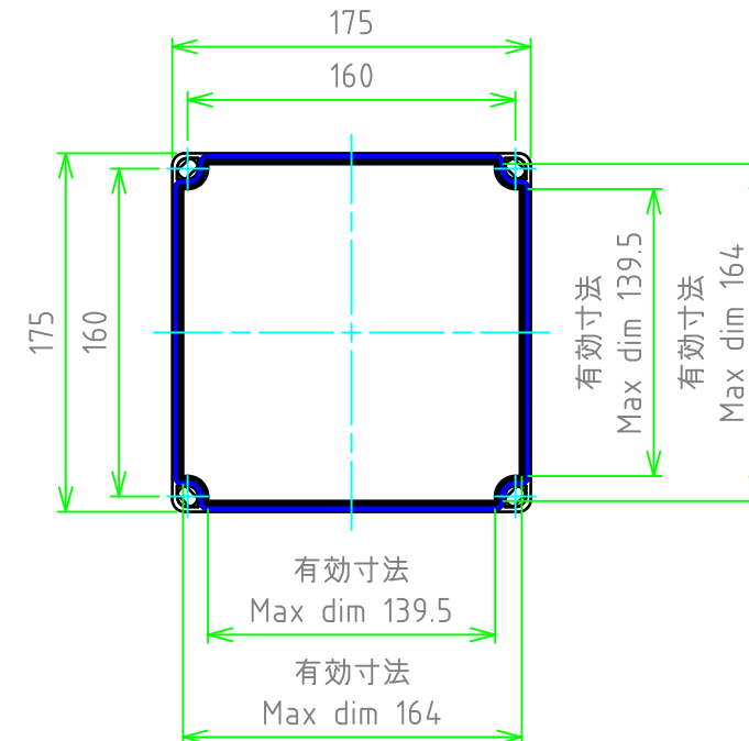
カバー(内視) Cover (Internal View)
