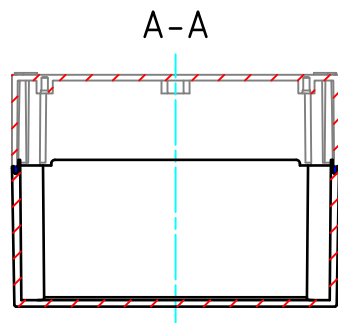
ボディー(内視) Base (Internal View)
