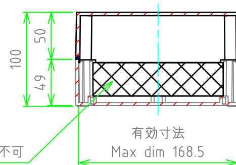
B-B
