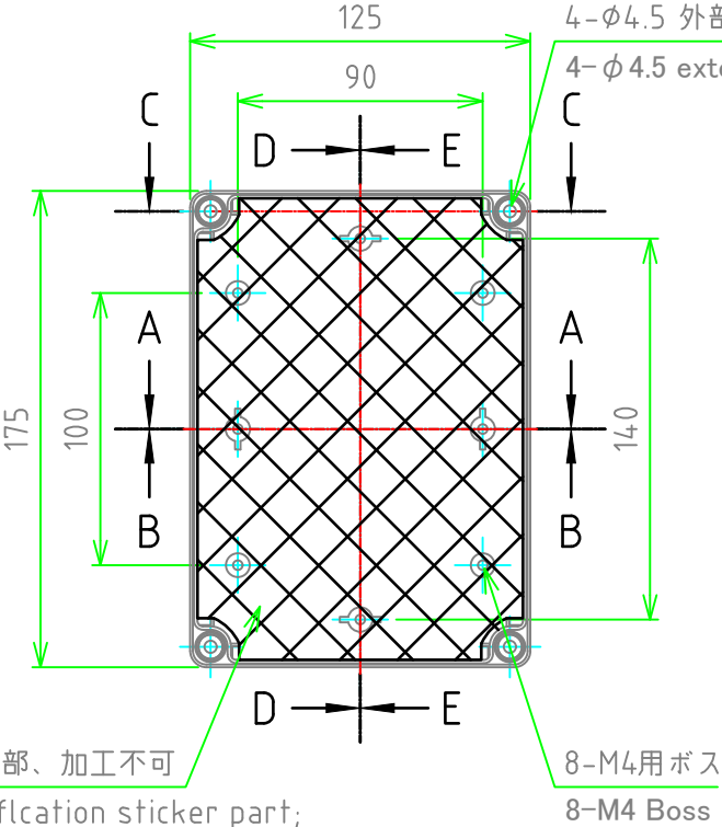
ボディー(内視) BASE (Internal View)
