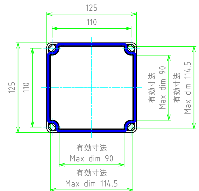
カバー(内視) Cover (Internal View)
