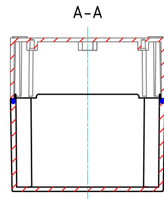
ボディー(内視) BASE (Internal View)
