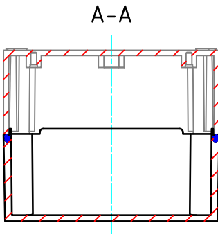
ボディー(内視) BASE (Internal View)
