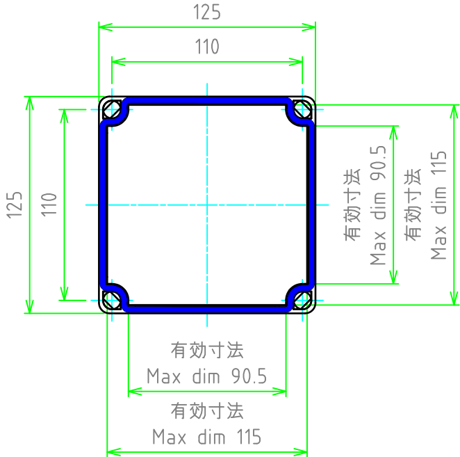
カバー(内視) Cover (Internal View)
