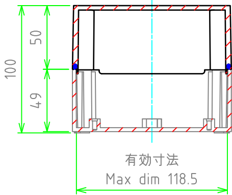
B-B
