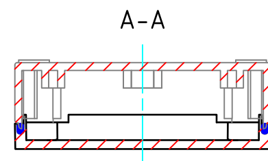
ボディー(内視) BASE (Internal View)
