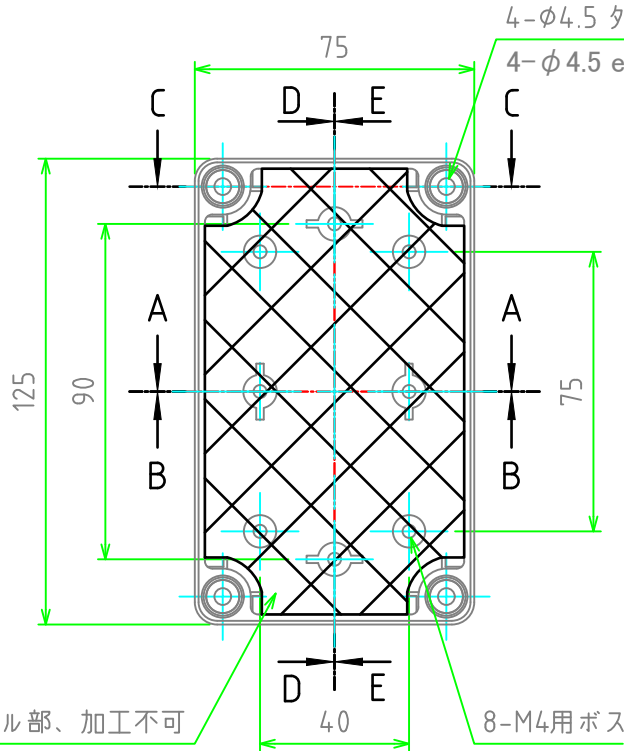
ボディー(内視) Base (Internal View)
