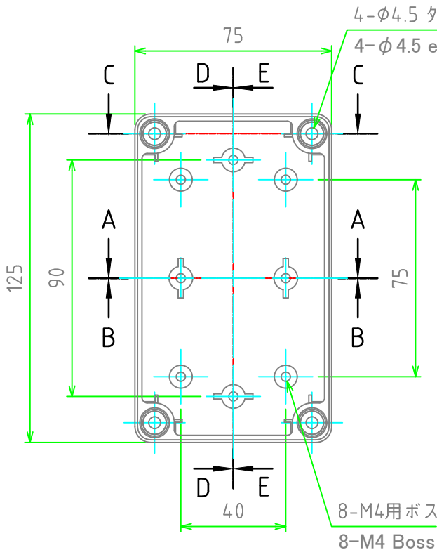
ボディー(内視) Base (Internal View)
