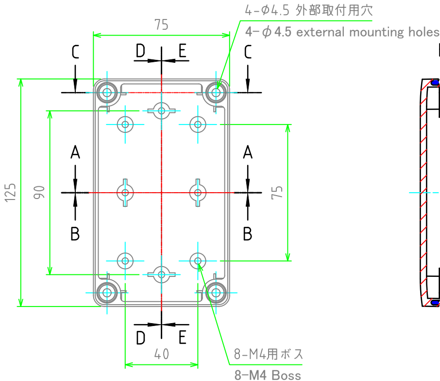
ボディー(内視) Base (Internal View)
