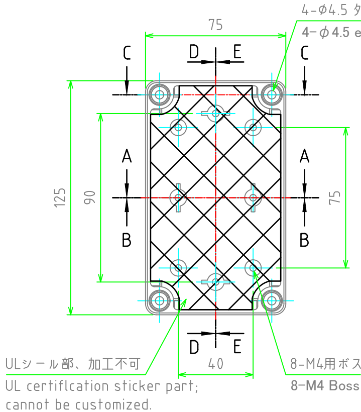
ボディー(内視) Base (Internal View)
