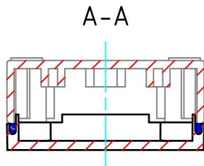
ボディー(内視) Base (Internal View)
