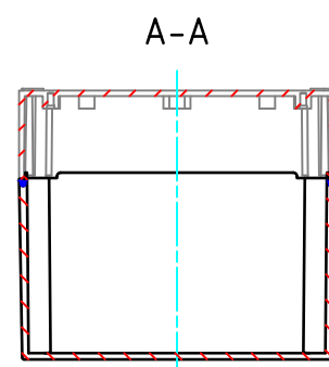
ボディー(内視) Base (Internal View)
