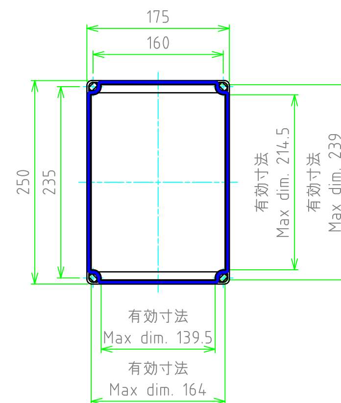
カバー(内視) Cover (Internal View)
