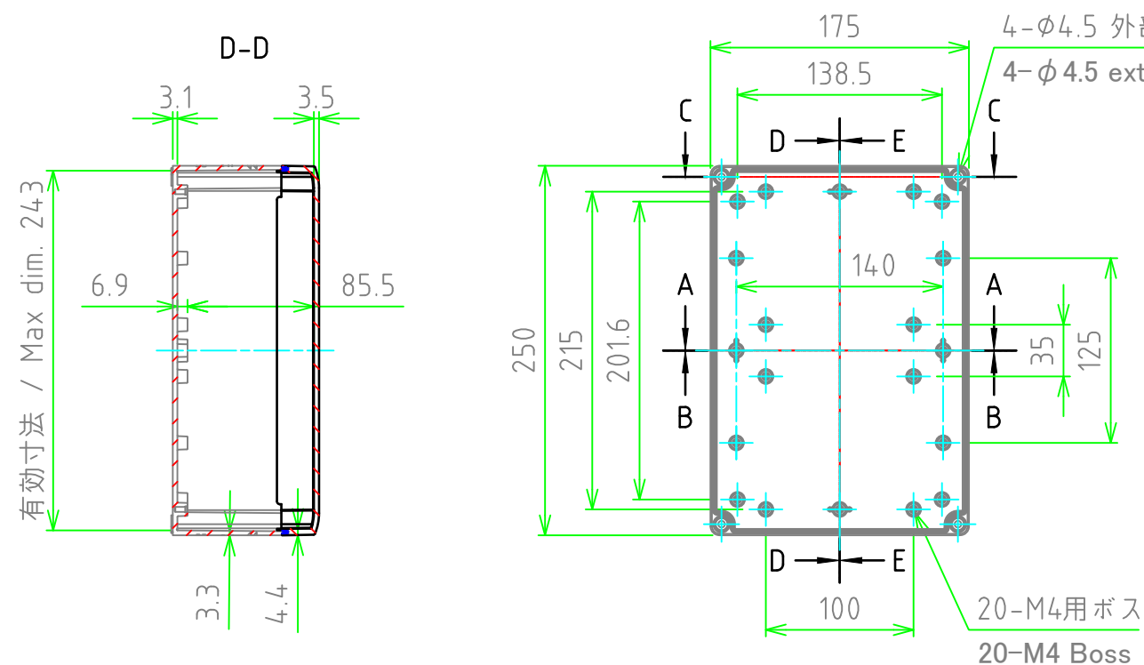
ボディー(内視) Base (Internal View)
