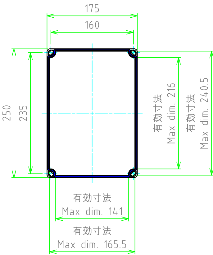
カバー(内視) Cover (Internal View)
