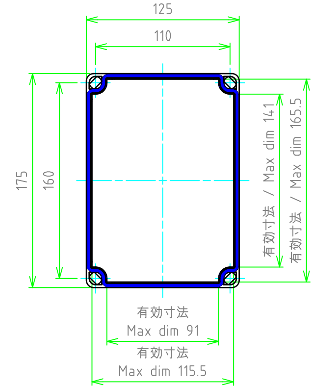
カバー(内視) Cover (Internal View)
