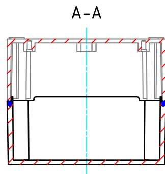
ボディー(内視) BASE (Internal View)
