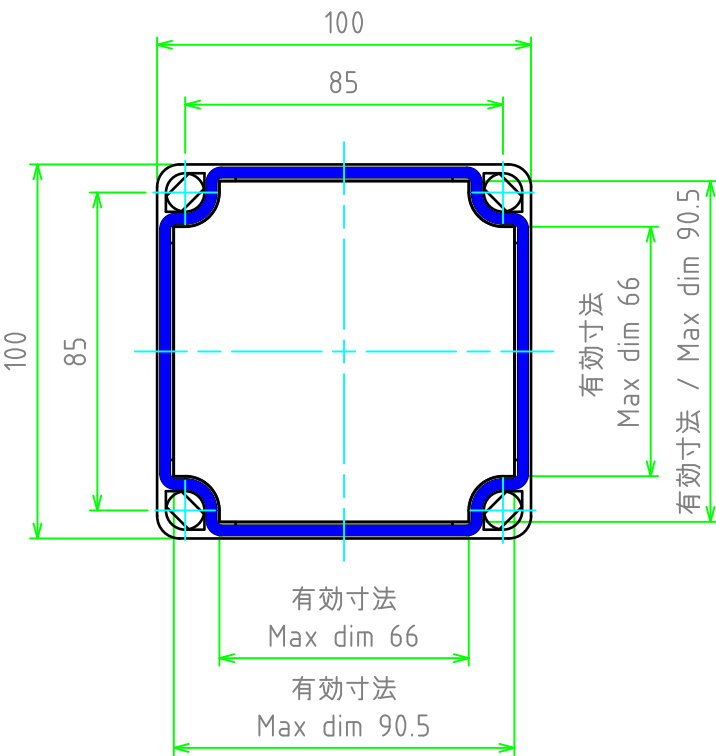
カバー(内視) Cover (Internal View)
