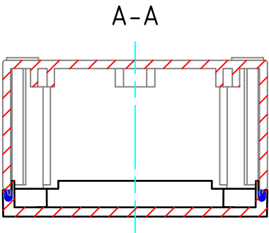
ボディー(内視) BASE (Internal View)
